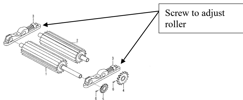
Figura n.10 adjustable roller
